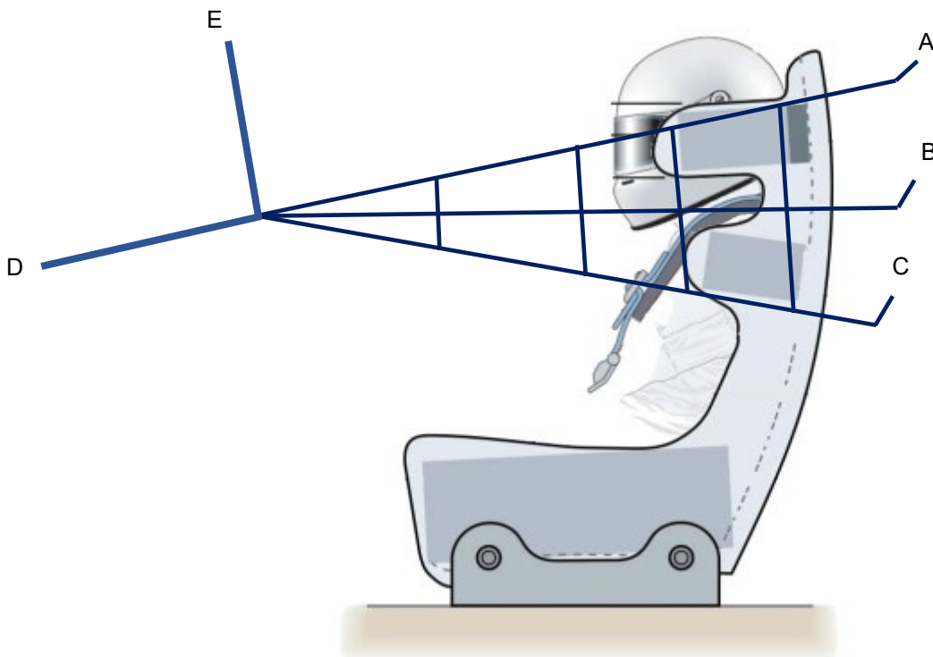
Figure 3. Position recommandée pour la tête et les épaules des pilotes par rapport au filet de course Figure 3. Recommended position of the driver's head and shoulder relative to the racing net
